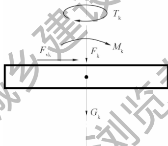
图 4.1.1 基础荷载
