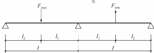
图 6.4.5-2 暗梁 (1-1 截面) 计算简图
