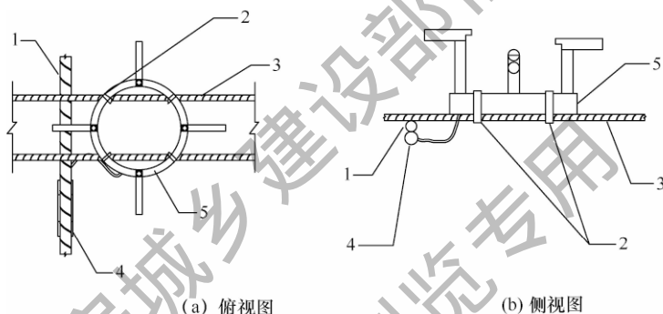
图 8.3.1 预埋式锈蚀传感器安装示意
